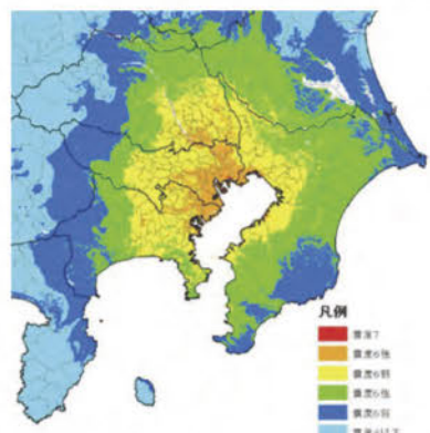
図1 震度分布(都心南部直下地震)※
